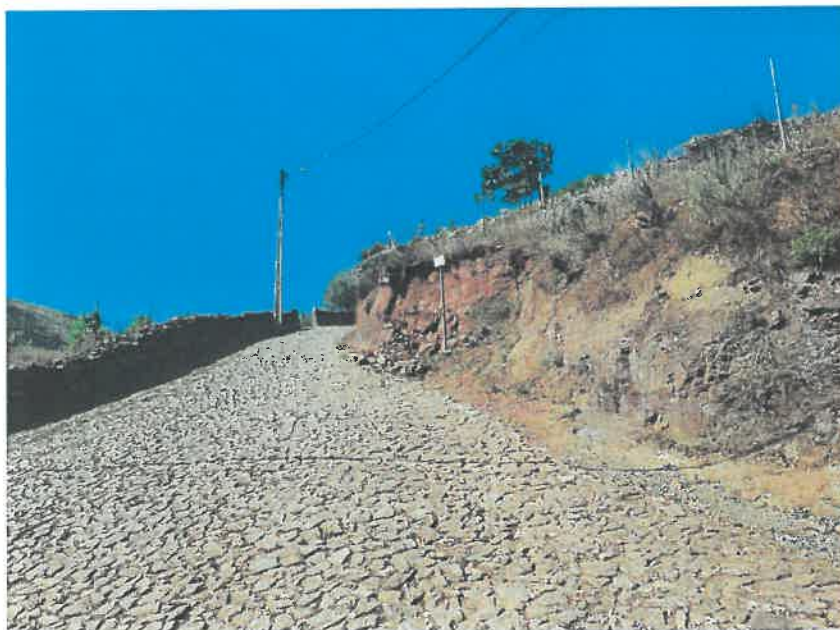
Figura 32 – Rua do Tubeiro de Cima. Instabilização do talude de escavação.
